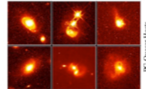
(f) Quasar
