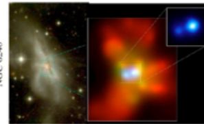
(d) Coalescence/(U)LIRG
